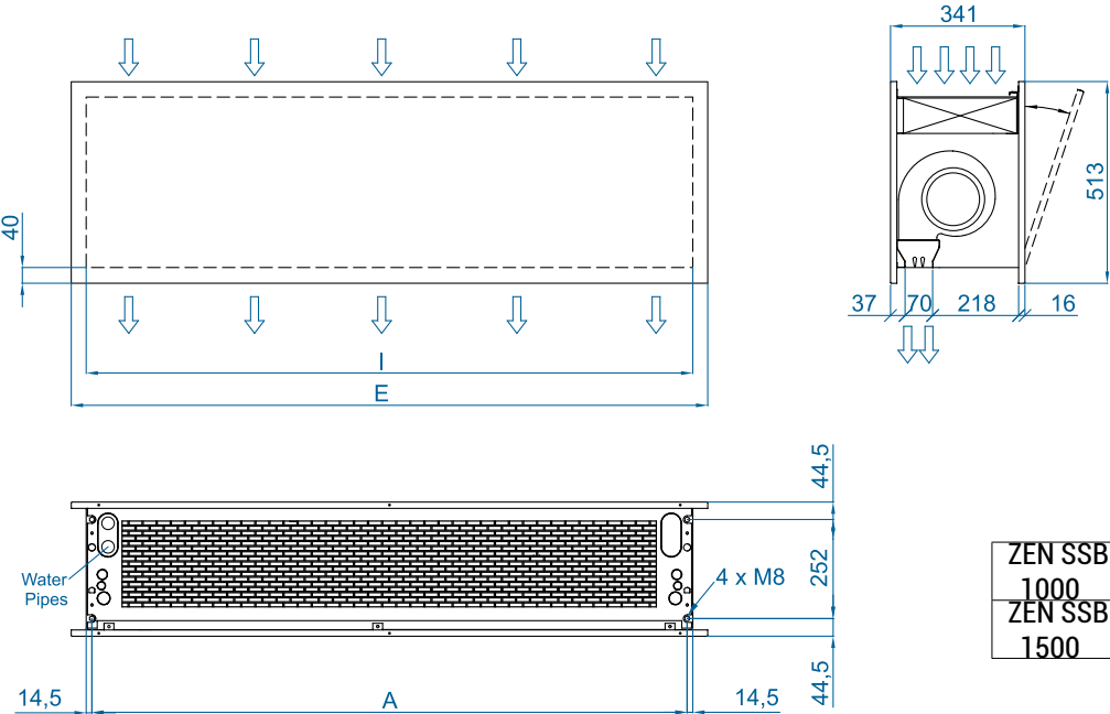
Instal·lació horitzontal
