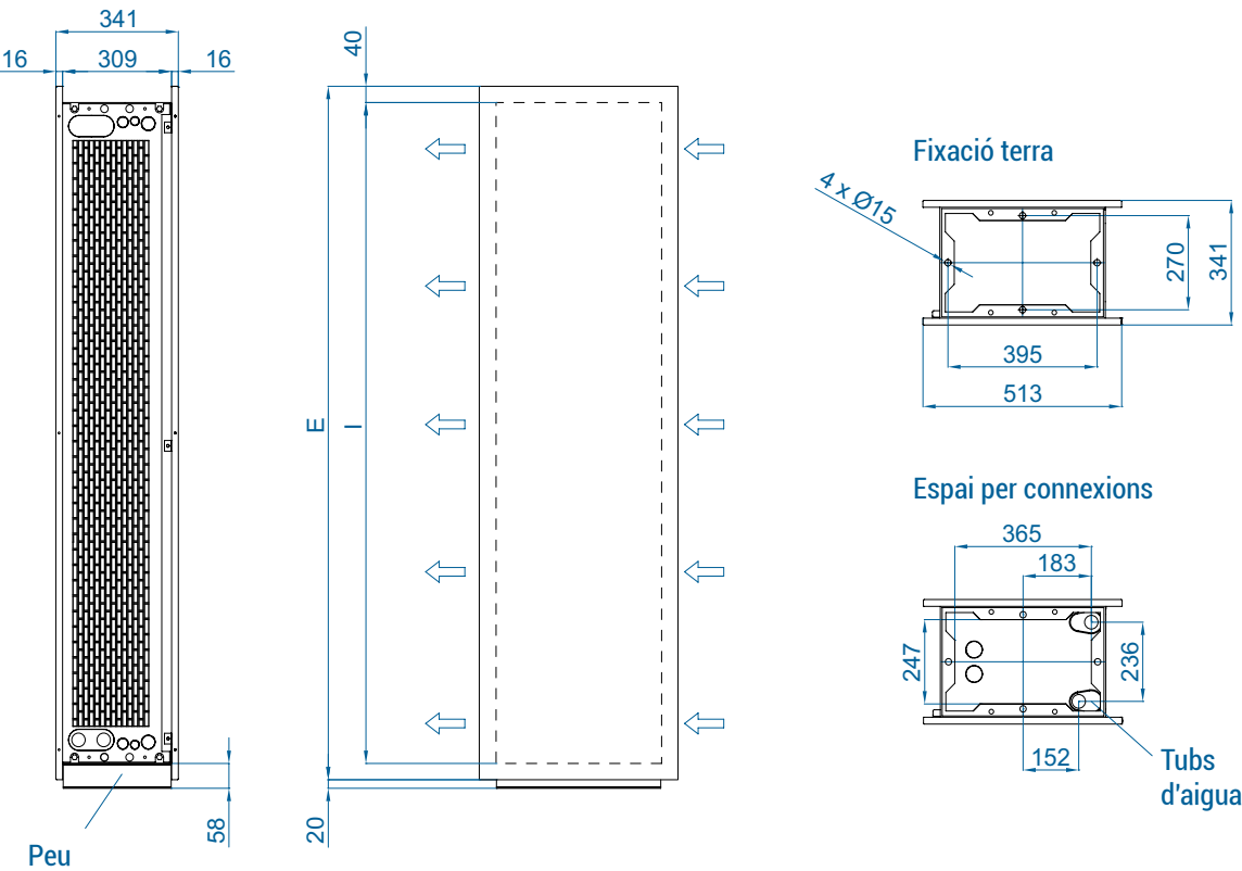
Instal·lació vertical
