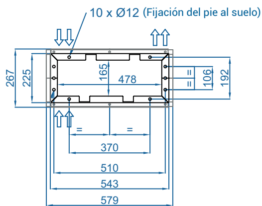
(Fijación del pie al bastidor)
